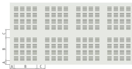
A = 78,5 / B = 440 / C = 160 mm % Perforación: 10,7
