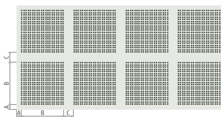
A = 55 / B = 487 / C = 113 mm % Perforación: 16
