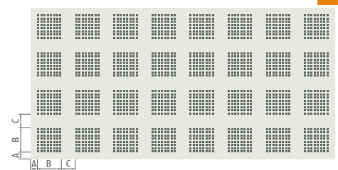
A = 55 / B = 187 / C = 113 mm % Perforación: 10,3
