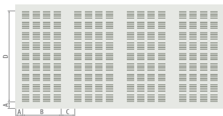
A = 78,5 / B = 440 / C = 160 / D = 1040 mm % Perforación: 12,1
