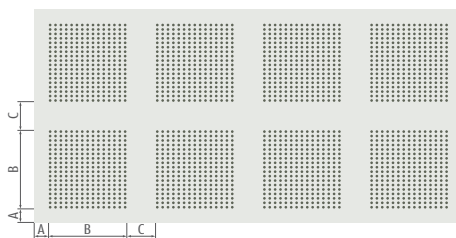
A = 81 / B = 435 / C = 165 mm % Perforación: 11,1
