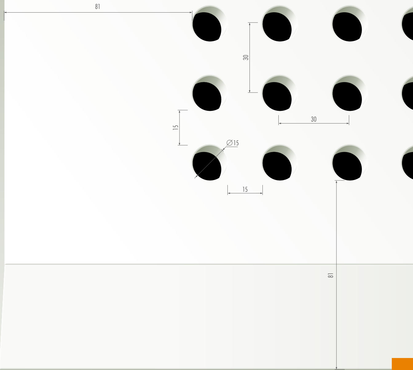
Imagen escala 1:1 Cotas en mm.
