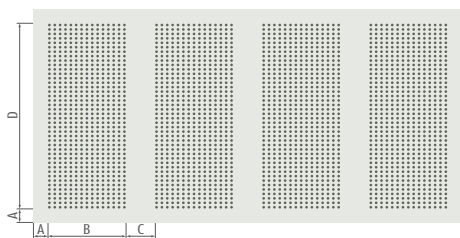
A = 81 / B = 435 / C = 165 / D = 1035 mm % Perforación: 12,9
